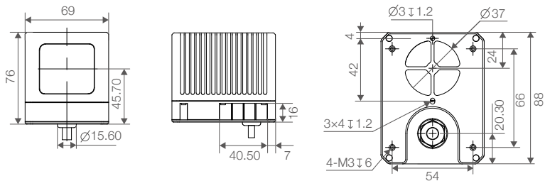
图 3.2.1 Livox Mid-40 尺寸结构（大图请查看附录 1）
